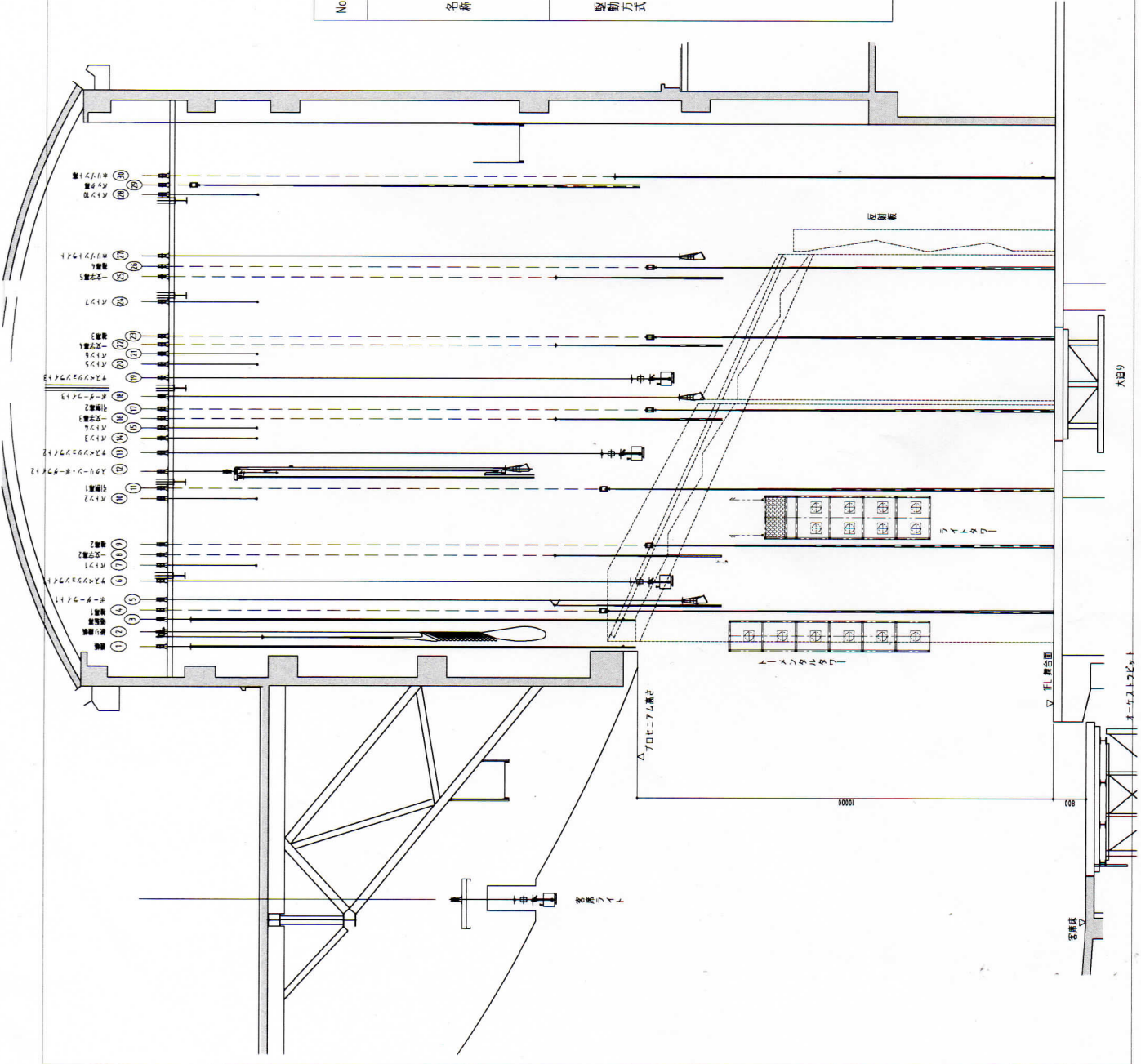
大府市勤労文化会館 もちのきホール 舞台吊物装置断面図
